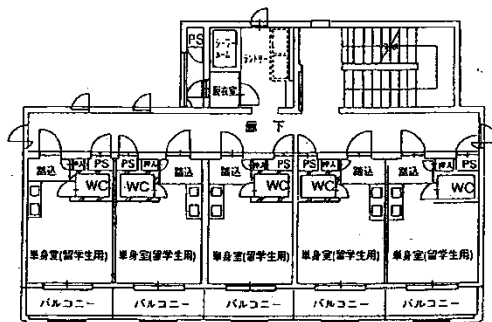
2～4階平面図
