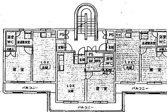
3・4 階平面図
