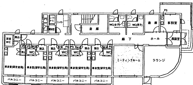
1階平面図
