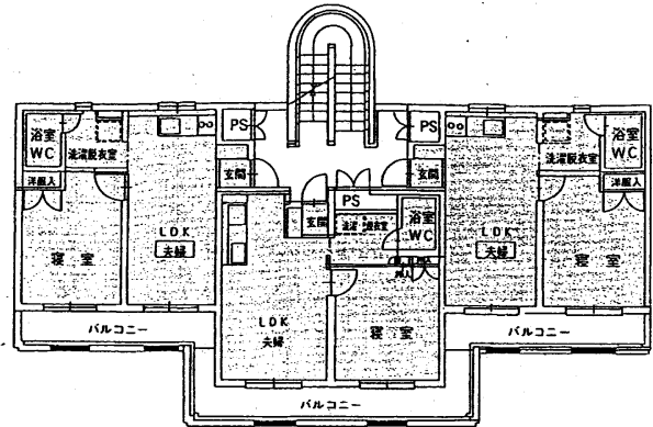
3・4階平面図
