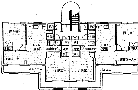
1・2階平面図
