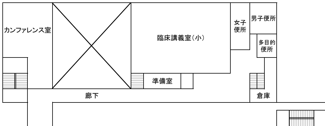
臨床講義棟 1階平面図
