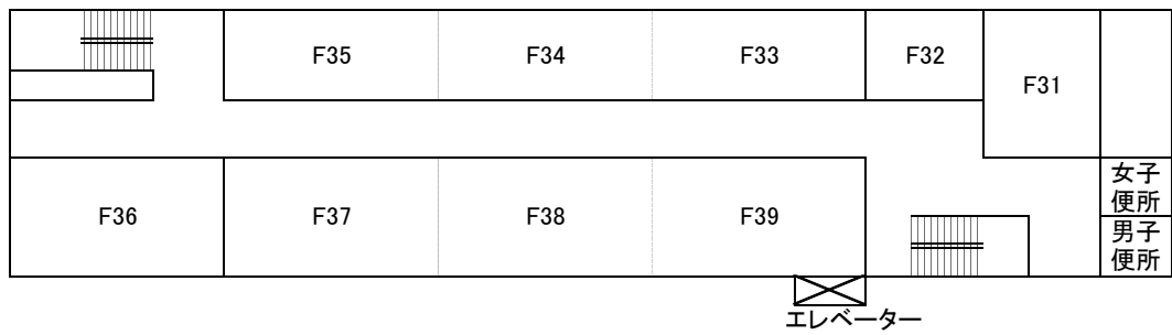
福利施設棟 3階平面図
