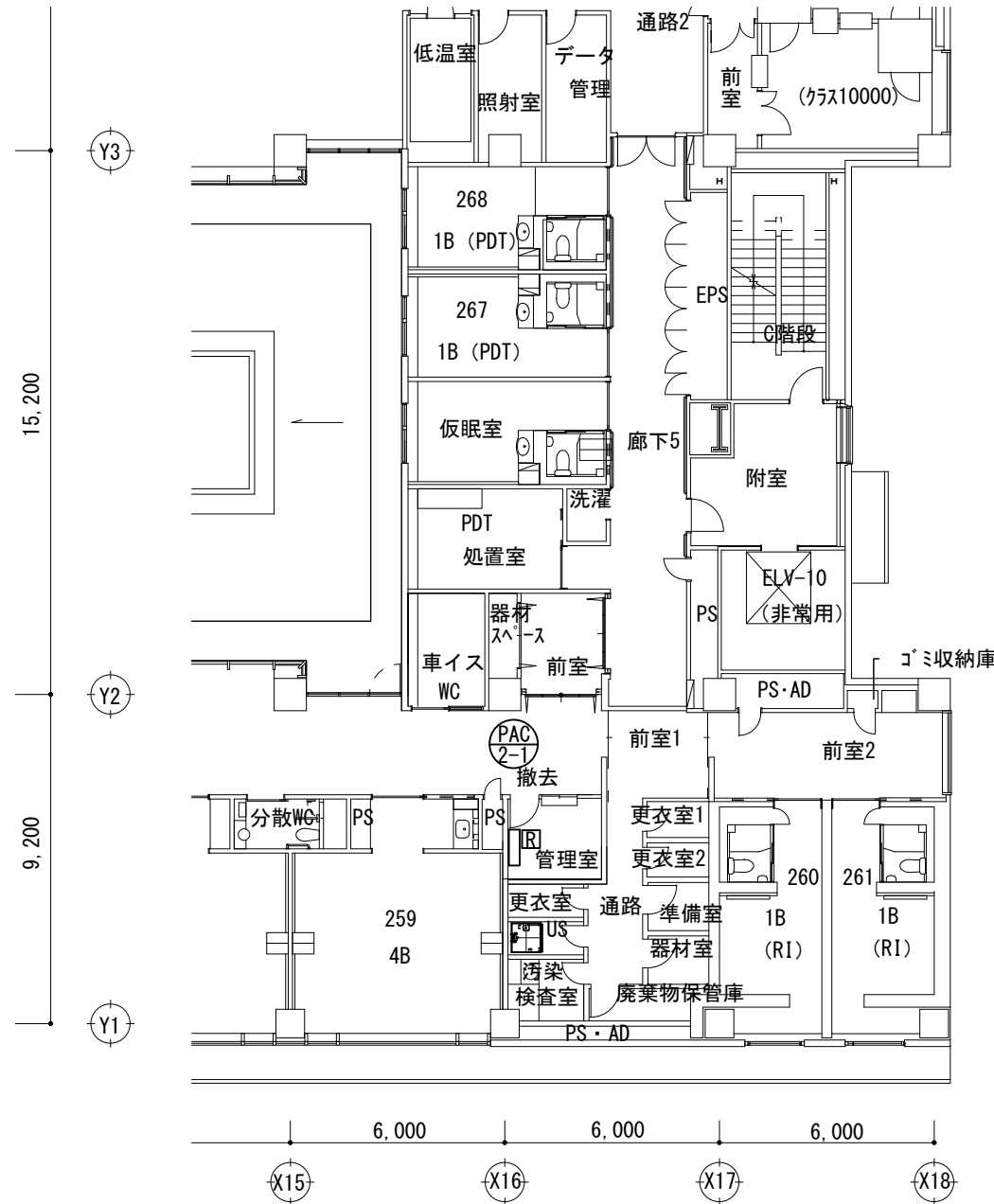
病棟2階空調撤去図 S=1/200
