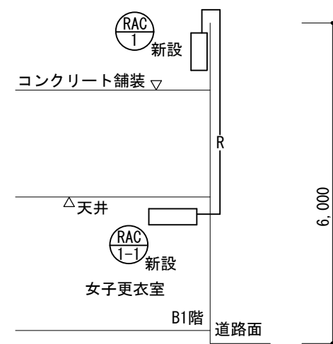
外来棟空調改修図(断面) S=1/100
