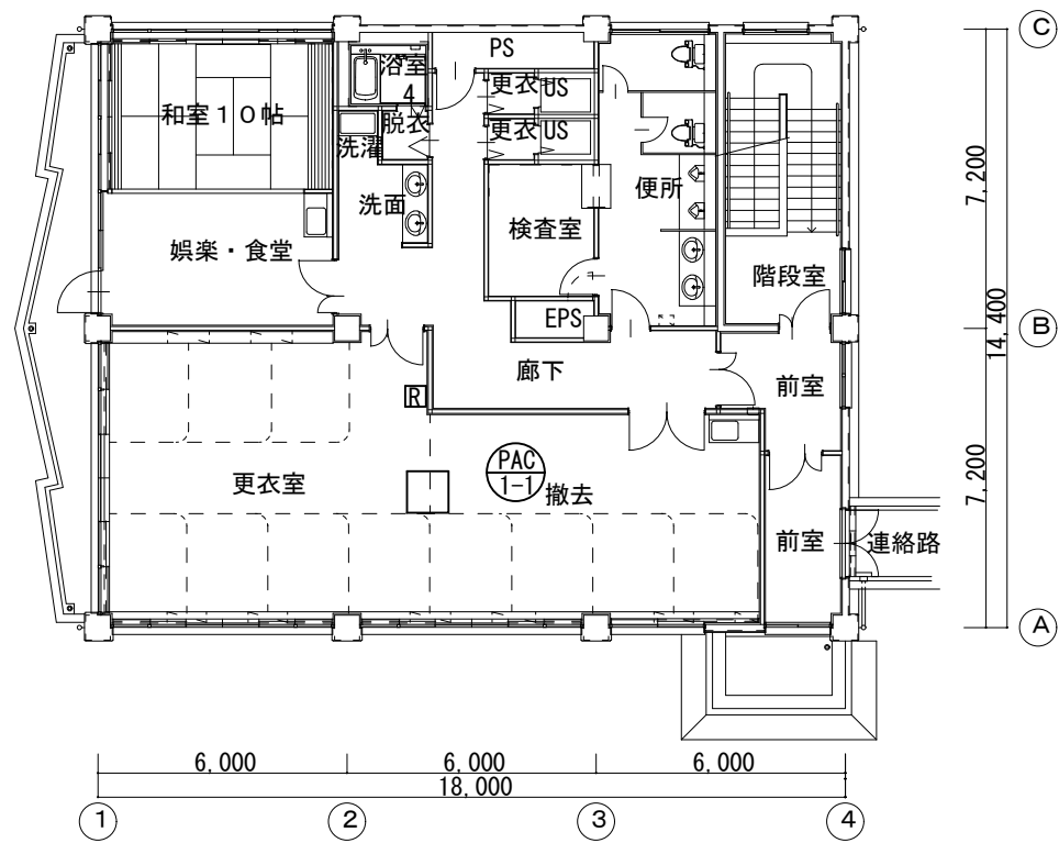
探索的臨床研究施設2階空調撤去図 S=1/200
