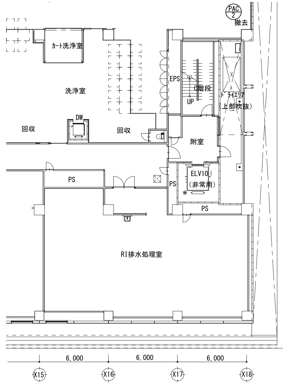
病棟地下1階空調撤去図 S=1/200
