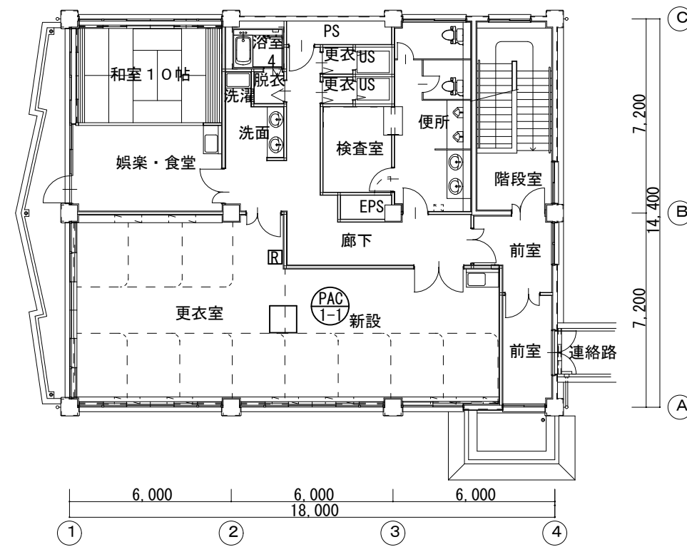
探索的臨床研究施設2階空調改修図 S=1/200
