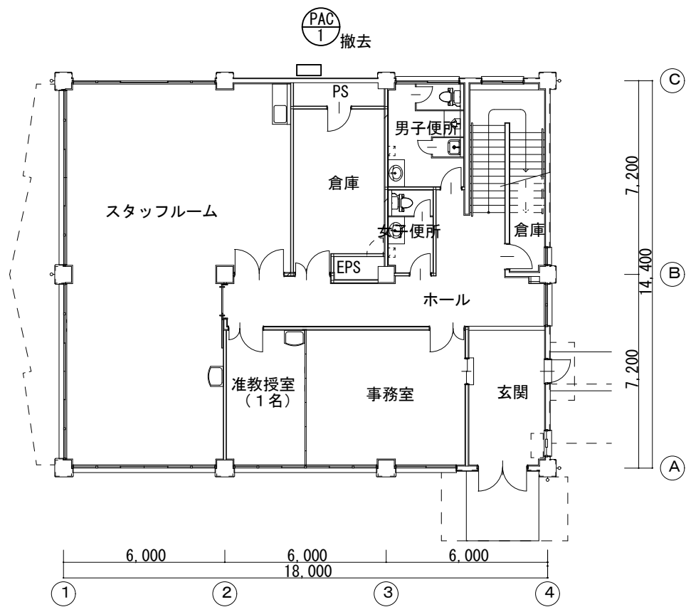
探索的臨床研究施設1階空調撤去図 S=1/200
