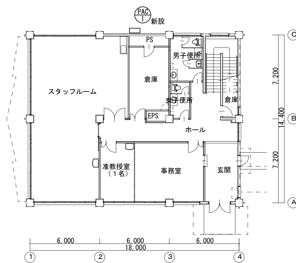
探索的臨床研究施設1階空調改修図 S=1/200
