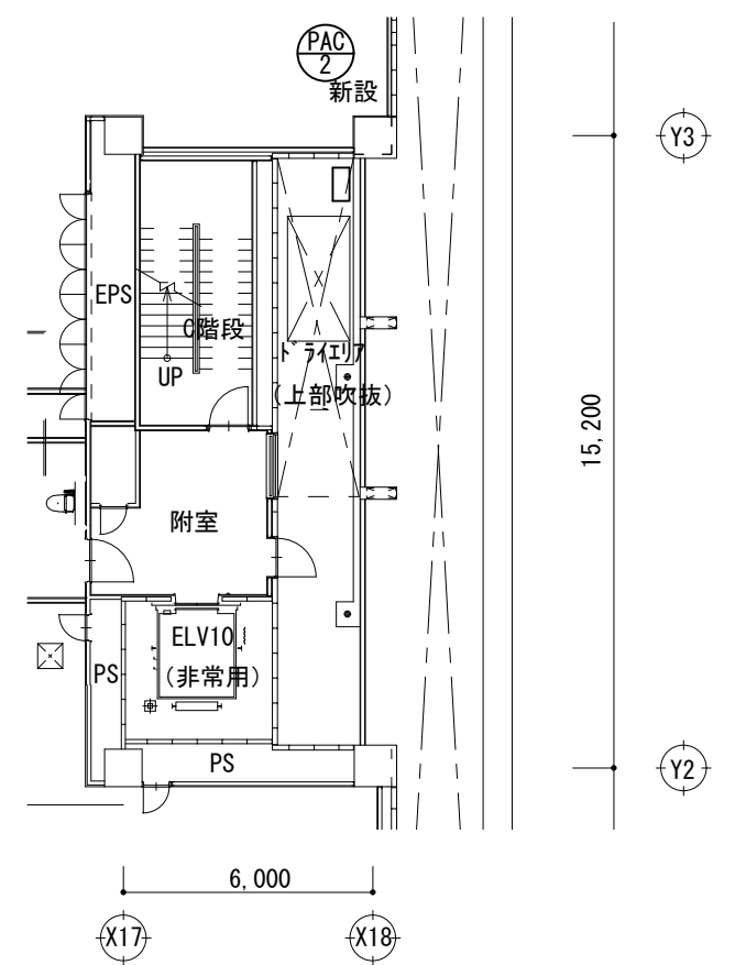
病棟地下1階空調改修図 S=1/200
