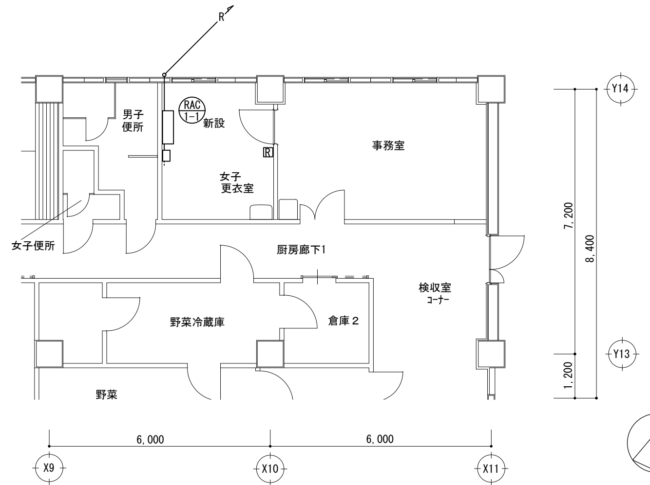
外来棟地下1階空調改修図 S=1/100
