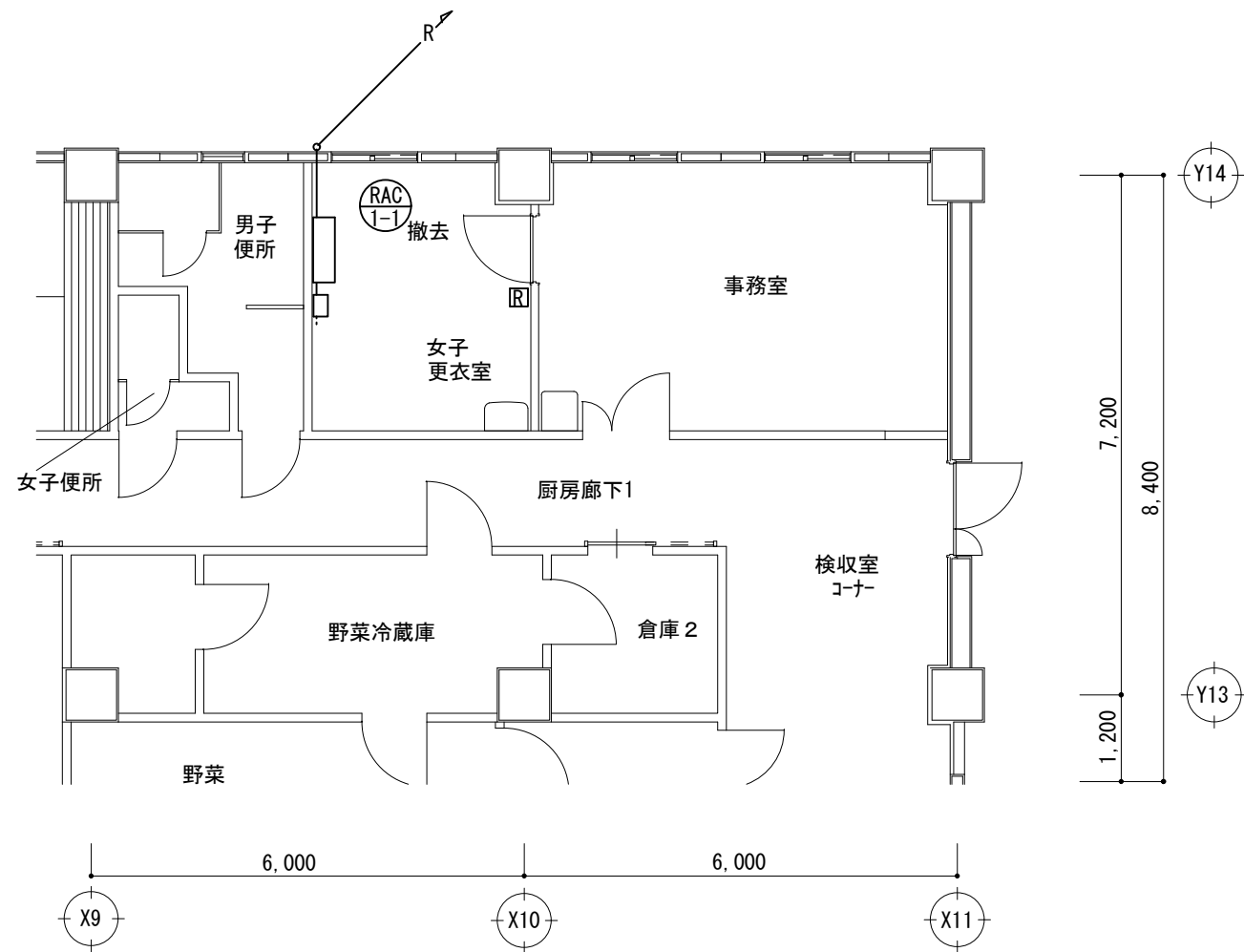
外来棟地下1階空調撤去図 S=1/100
