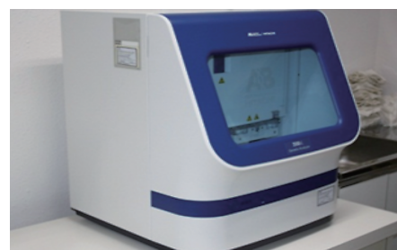
2 DNA シーケンサー
